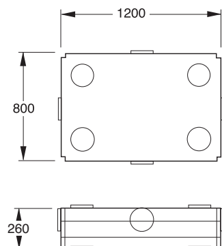
Kompakt-kassett
