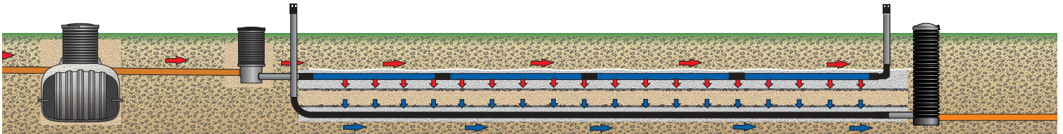
Septic III infiltration med markbädd
